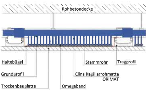
Deckenschnitt
